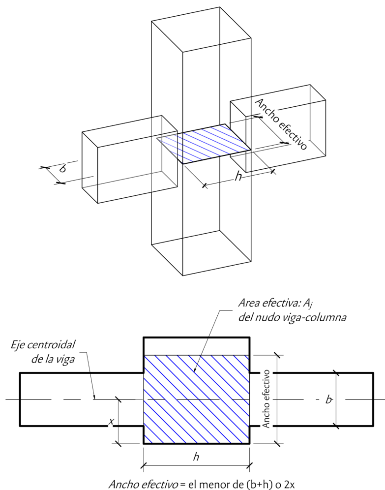
Figura 17: Área efectiva del nudo. Referencia: 5.12.1.10.4.
