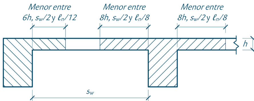
Figura 13: Geometría del ala efectiva en vigas T. Referencia: 5.9.8.
