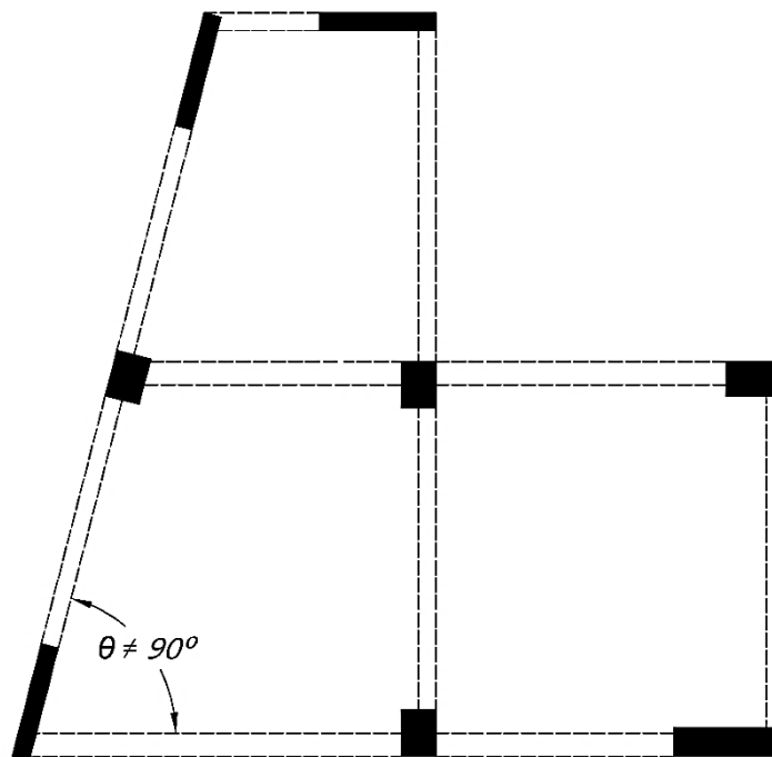
Figura 14. No ortogonalidad de los sistemas verticales sismorresistentes.
