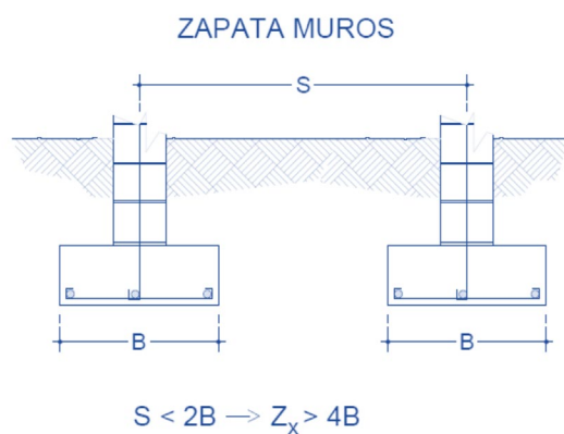
Figura 1: Espaciamento entre centros de columnas.
